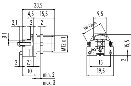
Leiterplattendicke: 1,6 mm Thickness of PCB: 1,6 mm Ansicht Bestückungsseite View of mating side
