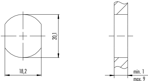
Schaltschrankdurchführung mit Durchgangsbohrung Lead-through for control cabinet with bore hole
