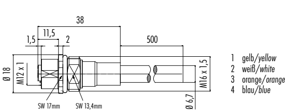
Maßzeichnung / Drawing
