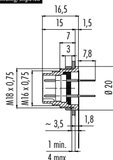
einreihig / Single-row
