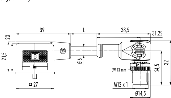
Maßzeichnung / Drawing
